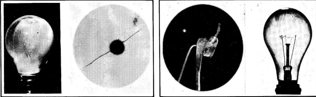
Las filtraciones de aire producen el blanqueamiento del vidrio. Si el filamento se afianza tan pobremente como se ilustra a la izquierda, la vida de la lámpara se acortará. A la derecha se el cristal de una lámpara importada dió origen a las grietas que se ilustran a la derecha.
