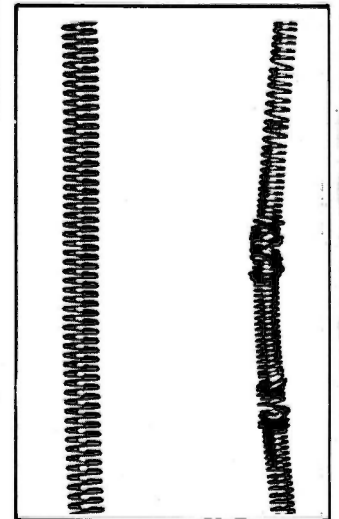
A la izquierda vemos, bastante agrandado, un filamento bueno; nótese la regularidad del espaciamiento. El filamento representado a la derecha fue encontrado en una lámpara barata.
